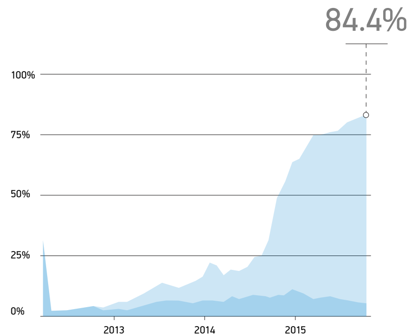
ПРОЦЕНТ ПОЛЬЗОВАТЕЛЕЙ МОБИЛЬНЫХ УСТРОЙСТВ С ПОДДЕРЖКОЙ WEBGL
