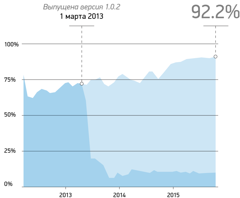
ПРОЦЕНТ ПОЛЬЗОВАТЕЛЕЙ ПЕРСОНАЛЬНЫХ КОМПЬЮТЕРОВ С ПОДДЕРЖКОЙ WEBGL
